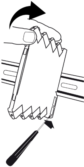
Figura 2: Smontaggio dalla guida DIN. Primo, ricordare di scollegare i connettori con voltaggi pericolosi. Staccare il dispositivo dalla guida DIN sollevando il blocco inferiore.
